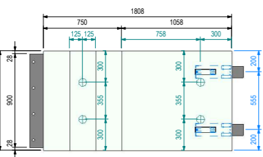
D Section D-D 1:25
